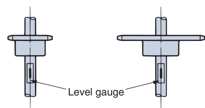
Fig. 15 Horizontal precision
